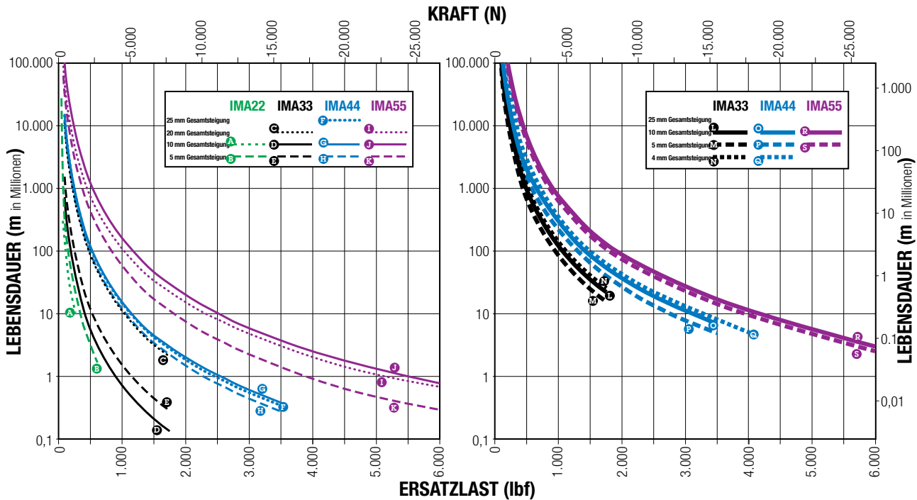
Alle Kurven stellen korrekt geschmierte und gewartete Antriebe dar.
